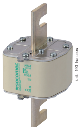
Fusible tipo aM, NH4 De 630 a 1250 A
